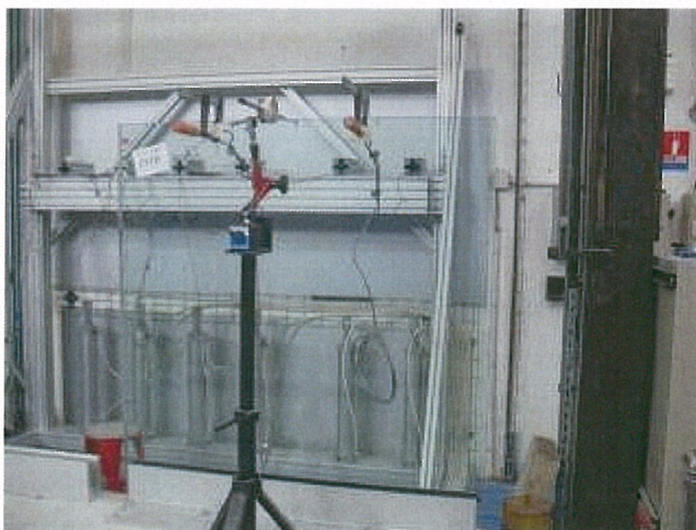
40 daN pendant 1 mn et 2 fois l'essai charge vers l'extérieur avec la charge statique pour le stade
