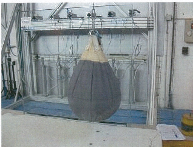
15 mn avec 3 fois la charge d'exploitation et choc mou au sac de 50 kg M50/700J
