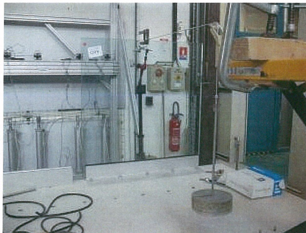
Mise en place de la cale à vitrage dans le profil et essai vers l'intérieur avec 20 daN pendant 3 mn.
