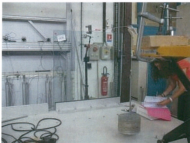
40 daN pendant 1 mn et 2 fois l'essai charge vers l'extérieur avec la charge statique pour le stade
