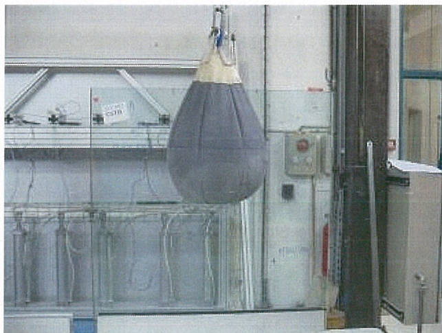
Essai de sécurité avec 3 fois la charge d'exploitation pendant 15 mn. Choc mou au sac M50/900J
