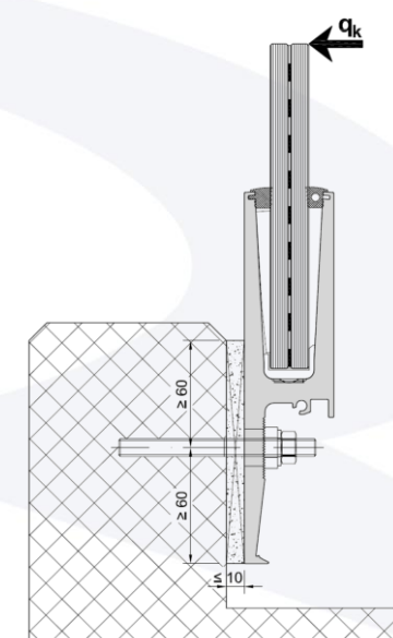
Abschränkung vor Brüstung
