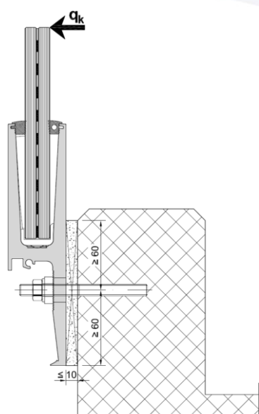
Abschränkung nach Brüstung / Stirne
