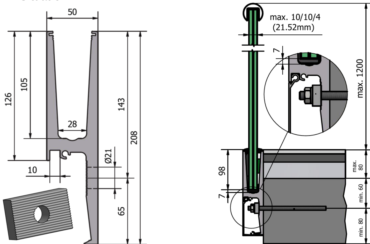
Schnitt Verglasungsschuh TL-3011 mit Klemmplatte und Geländer
