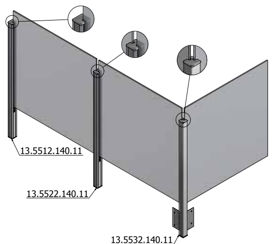
Seitenmontage für Handlauf
