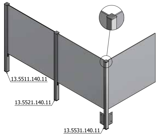
Seitenmontage oben offen
