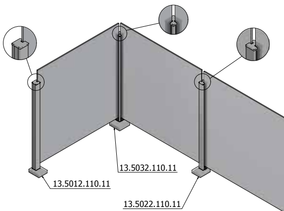
Bodenmontage oben offen
