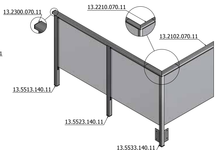
Seitenmontage für Handlauf
