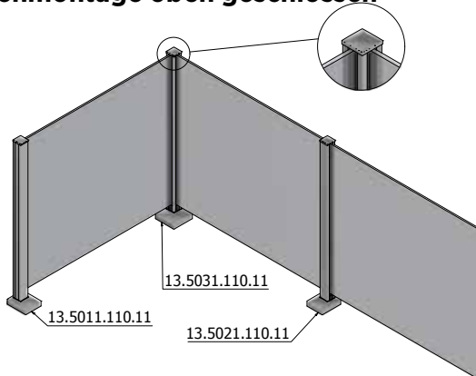
Bodenmontage oben geschlossen
