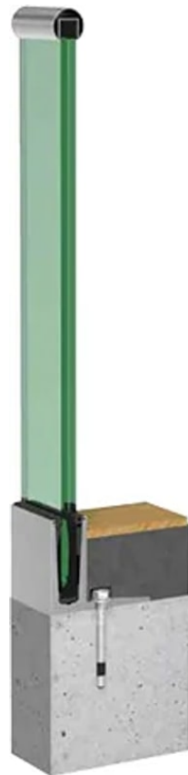
COUPE VERTICALE · GC-30
